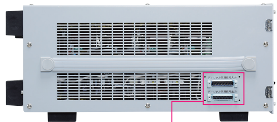
デジタル同期信号入力・出力
