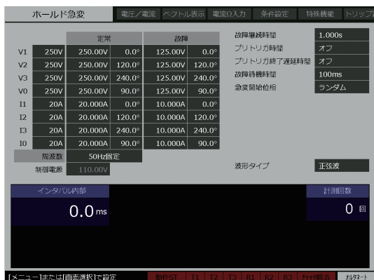
▲ホールド急変 メイン画面
