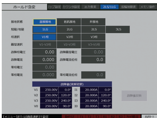
▲ホールド急変 2LS/1LG
