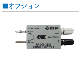
PA-001-2835 絶縁信号伝送アダプタ RX4744A / RX4744ASのトリップ入力とリクローズ入力のCOM端子間を電気的に絶縁
