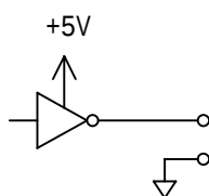
(a) TTL ロジック出力
