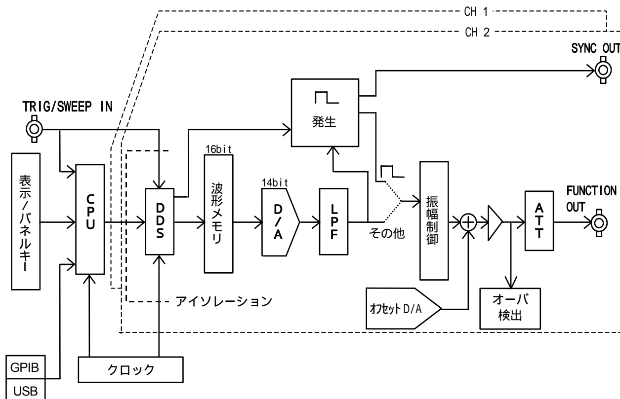
ブロック図
