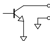
(b) オープンコレクタ出力
