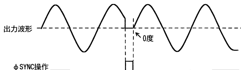
位相初期化操作と波形出力（位相＝0度のとき）
