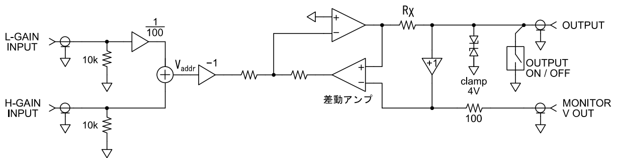
図 1-1 ブロック図
