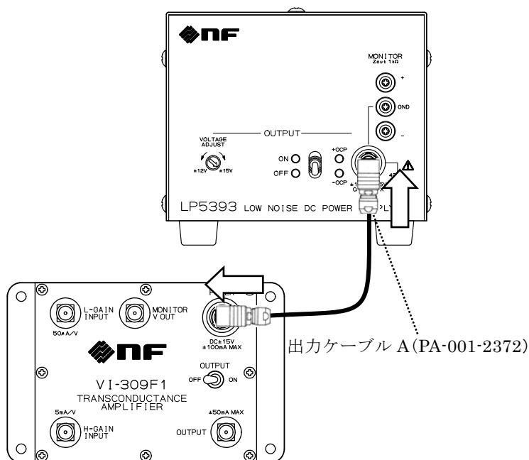
図 2-1 低雑音直流電源 LP シリーズとの接続
