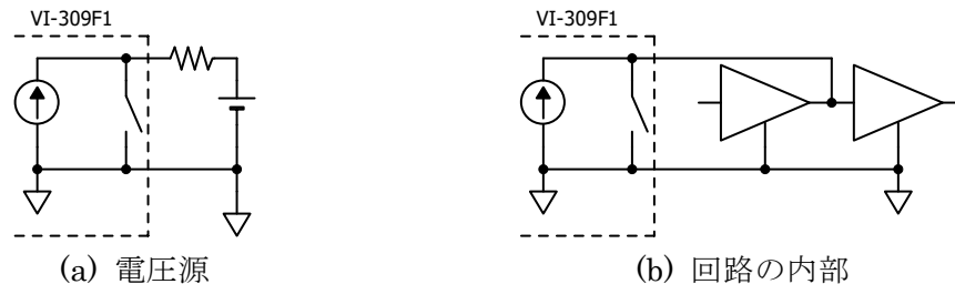
図 3-3 OUTPUT スイッチの使用に注意を要する負荷の例
