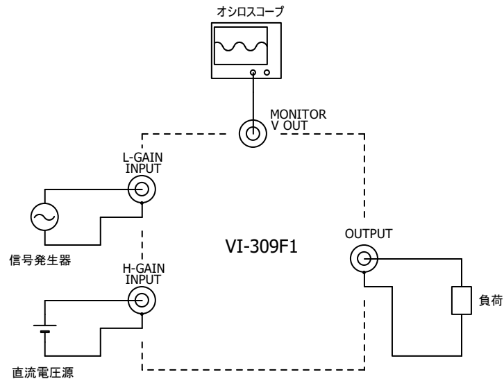
図 3-4 基本的な接続の例
