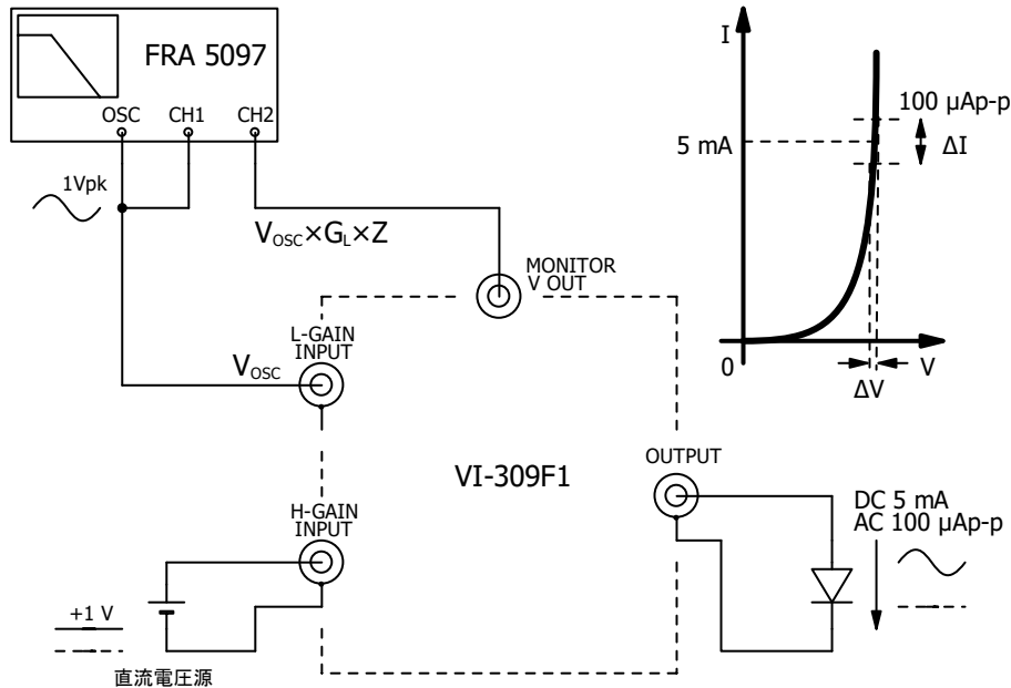
図 3-5 FRA との接続
