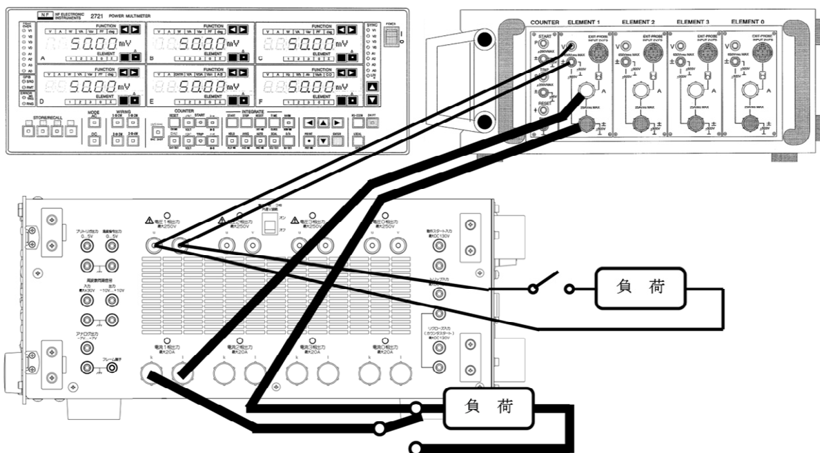
図 8-1 パワーマルチメータ（2721）と負荷の接続
