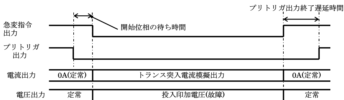
図 4-2 トランス突入電流模擬モードの試験シーケンスの例
