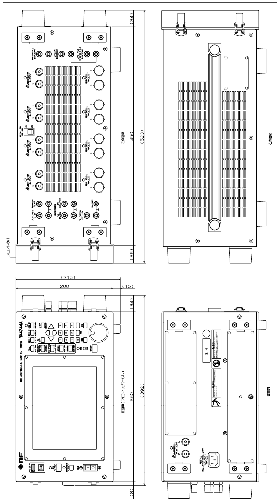
図 9-3 RX4744A 外形寸法図
