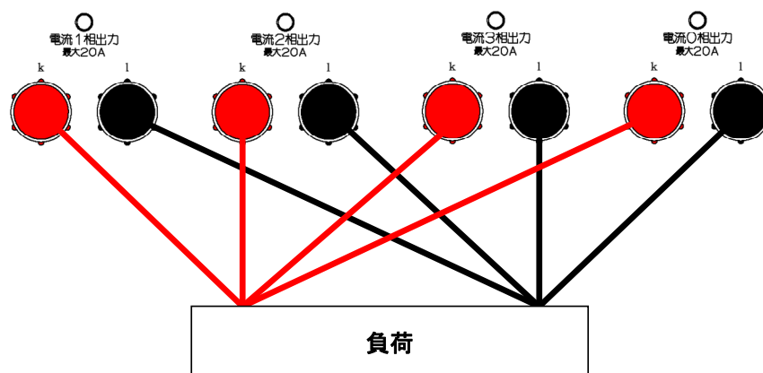
図 3-7 電流 4 並列の接続
