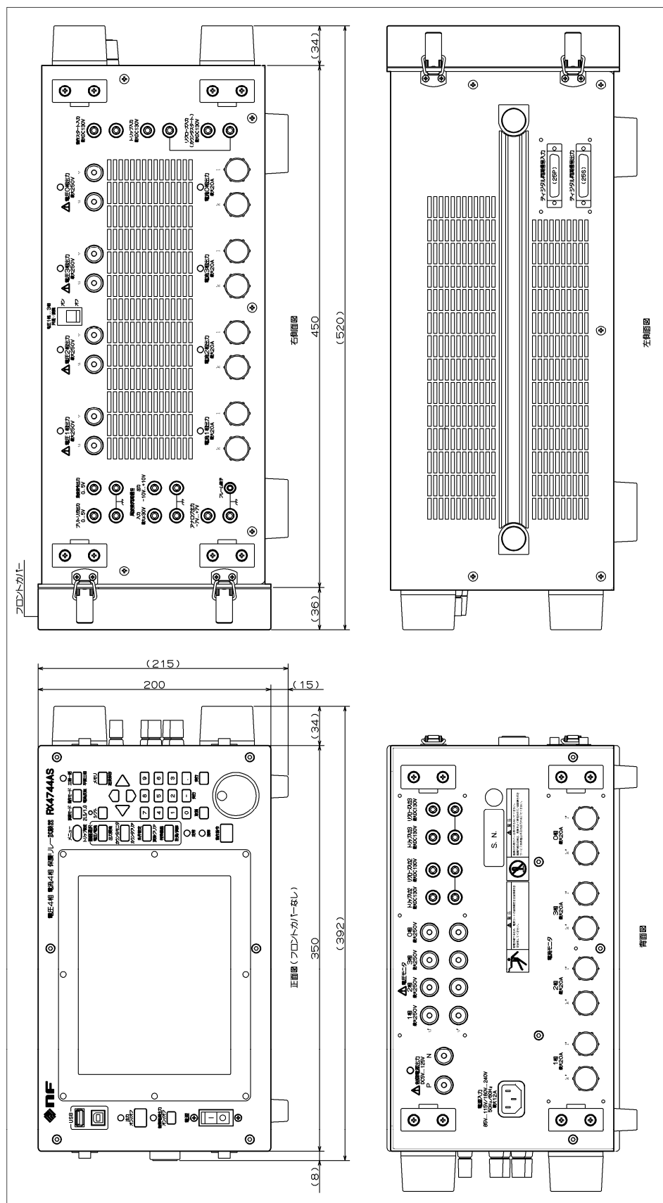
図 9-4 RX4744AS 外形寸法図
