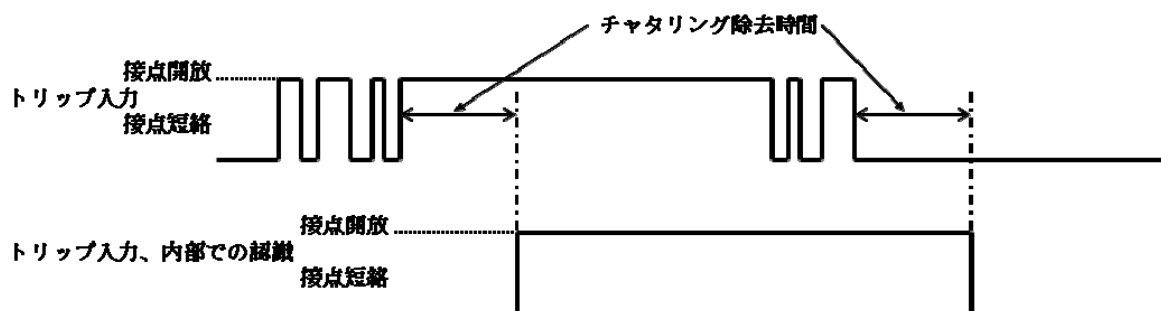
チャタリングしているトリップ信号（上）とチャタリング除去機能で認識したトリップ信号（下）
