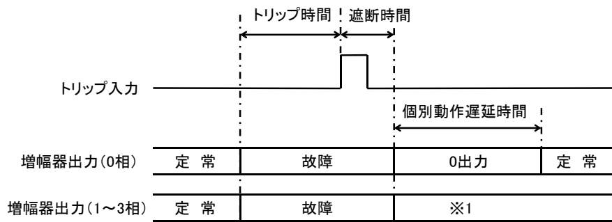
図 3-18 0 相動作を“個別”に設定したときの試験シーケンスの例
