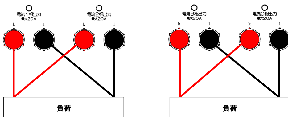
図 3-6 電流 2 並列の接続
