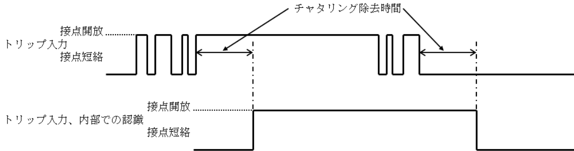
チャタリングしているトリップ信号（上）とチャタリング除去機能で認識したトリップ信号（下）
