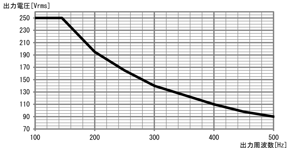
図 3-3 出力周波数と出力電圧
