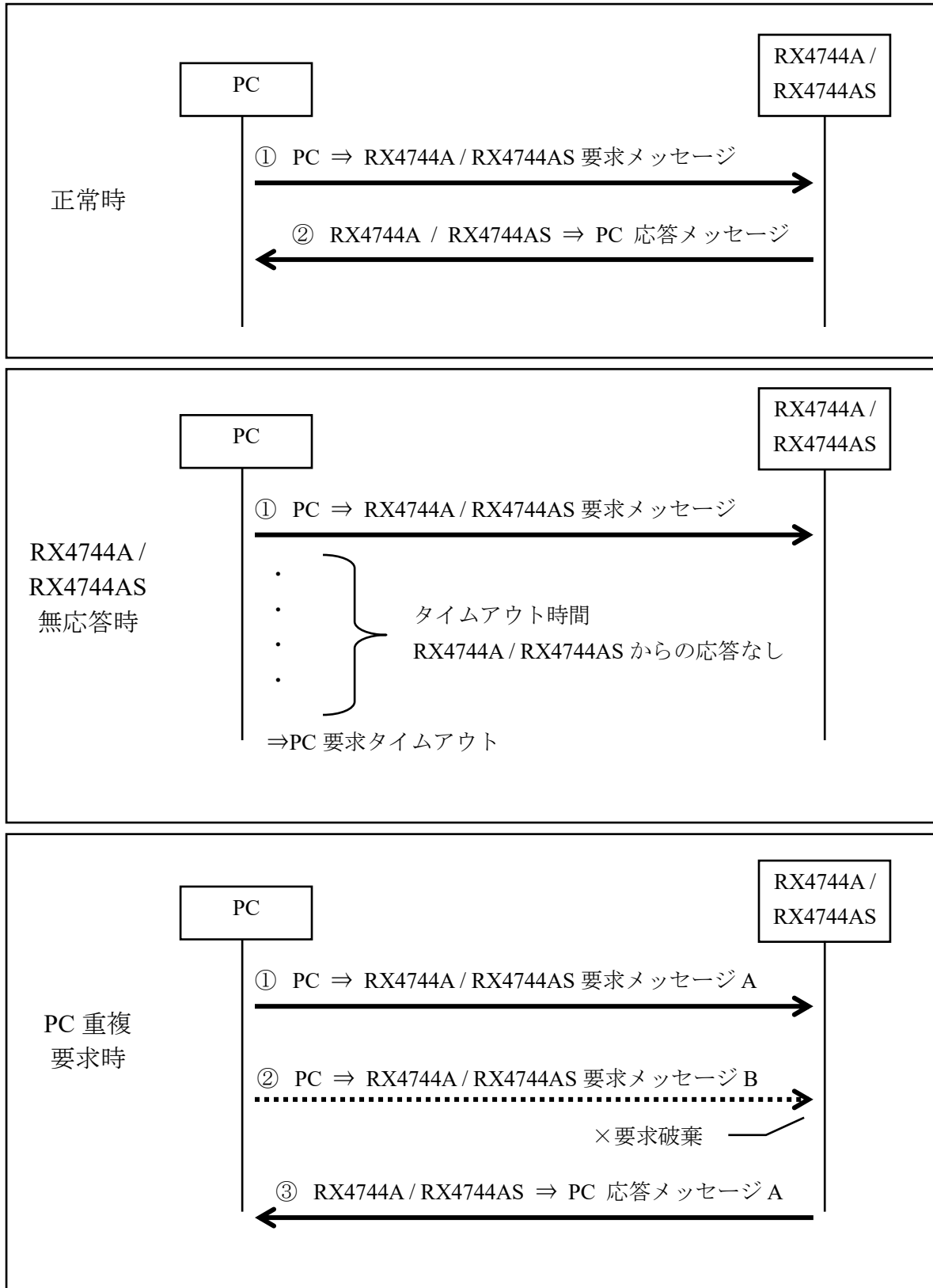
図 1-1 外部制御の通信手順イメージ
