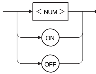
Figure 2.8 Boolean Value Parameter (<BOL>) Syntax
