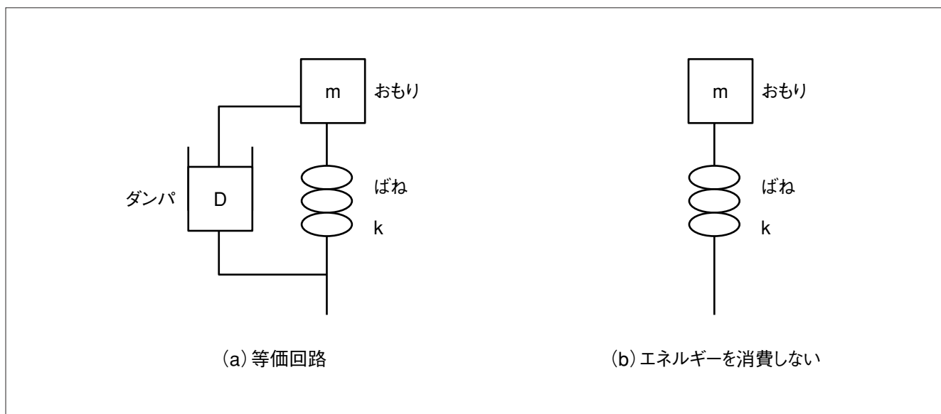
図2-2 センサの等価回路
