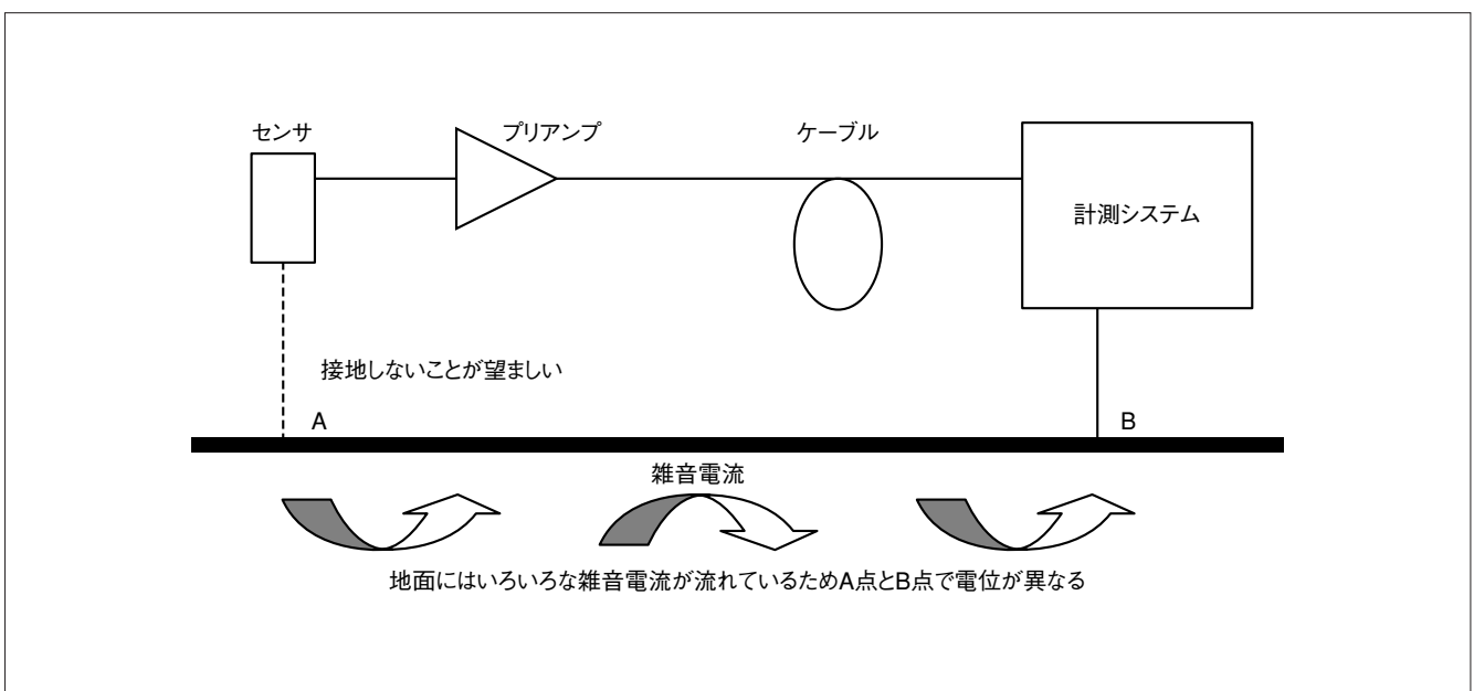
図2-7 接地
