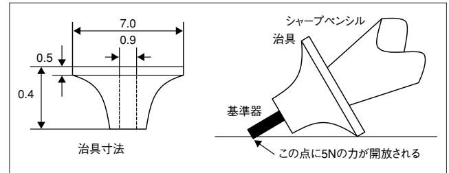
図2-5 シャープペンシル芯圧折法
