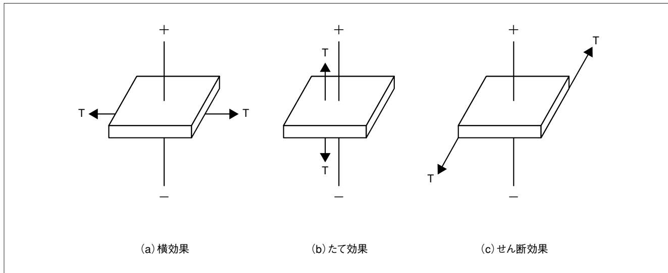
図2-1 圧電効果
