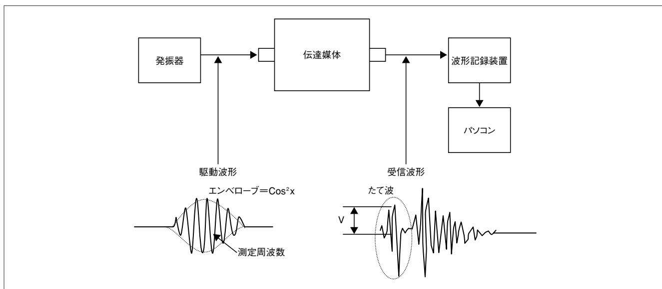
図2-3 相互校正法
