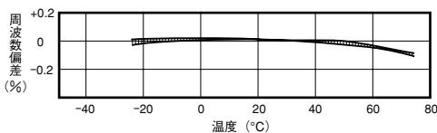
発振周波数温度特性 fo=100kHz
